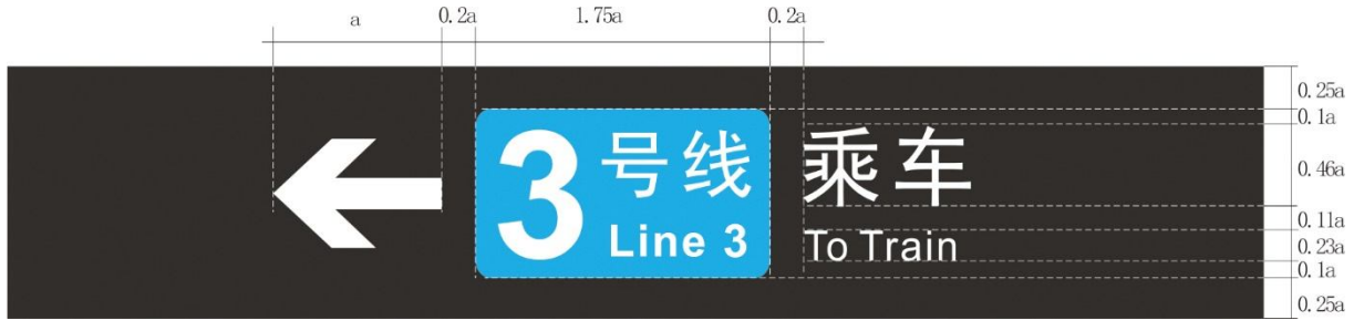
图13 单线线路标识与图形符号、文字规格示意图（站厅乘车导向标识）
