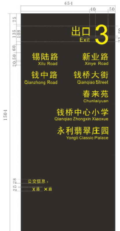
图52 出口信息标识
