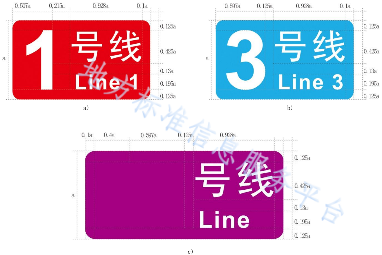
图9 线路标识中图形符号、文字规格示意图
