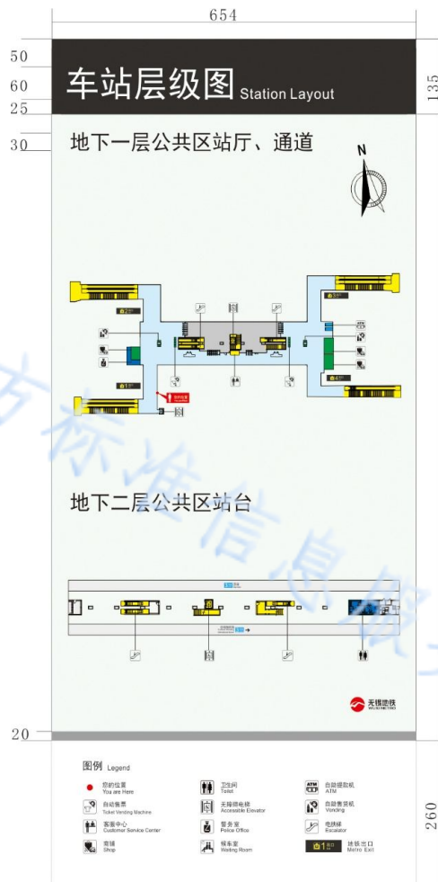
图51 车站层级图
