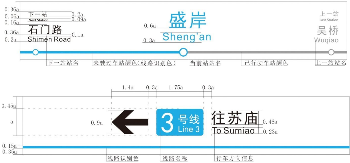
图41 列车运行方向导向标识
