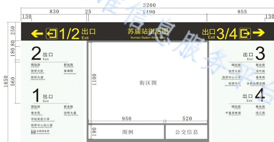
图46 站厅综合资讯柱贴标识
